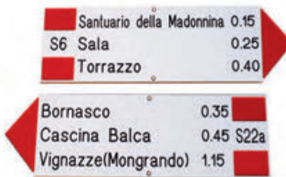
TARGA SEGNALETICA ART. 5810 HPL Incisa L 550 X H 150 mm
